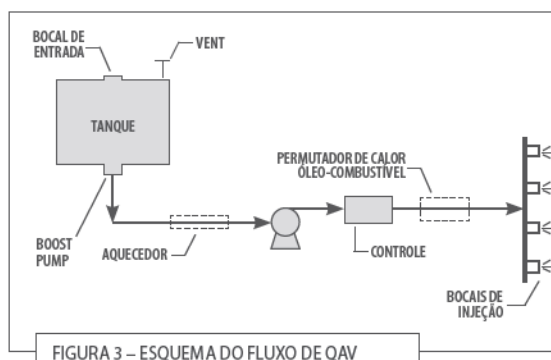
FIGURA 3 – ESQUEMA DO FLUXO DE QAV
