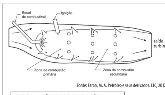
FIGURA 2 – CÂMARA DE COMBUSTÃO
